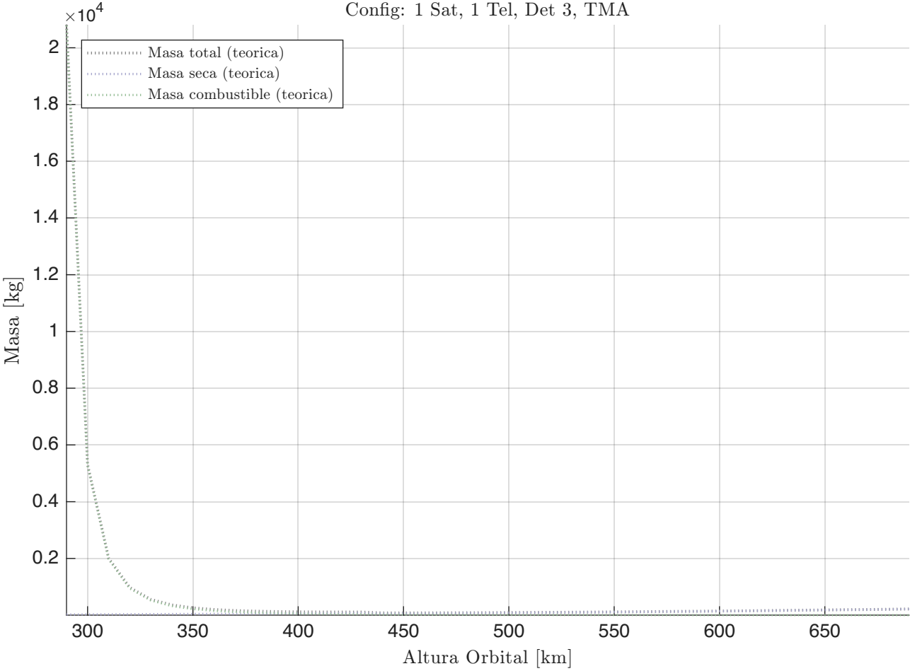
Desglose de Masas vs. Altura Config: 1 Sat, 1 Tel, Det 3, TMA
